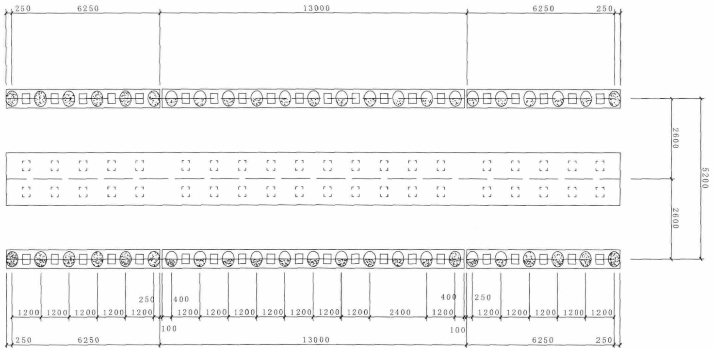
承台及千斤顶平面设计图
